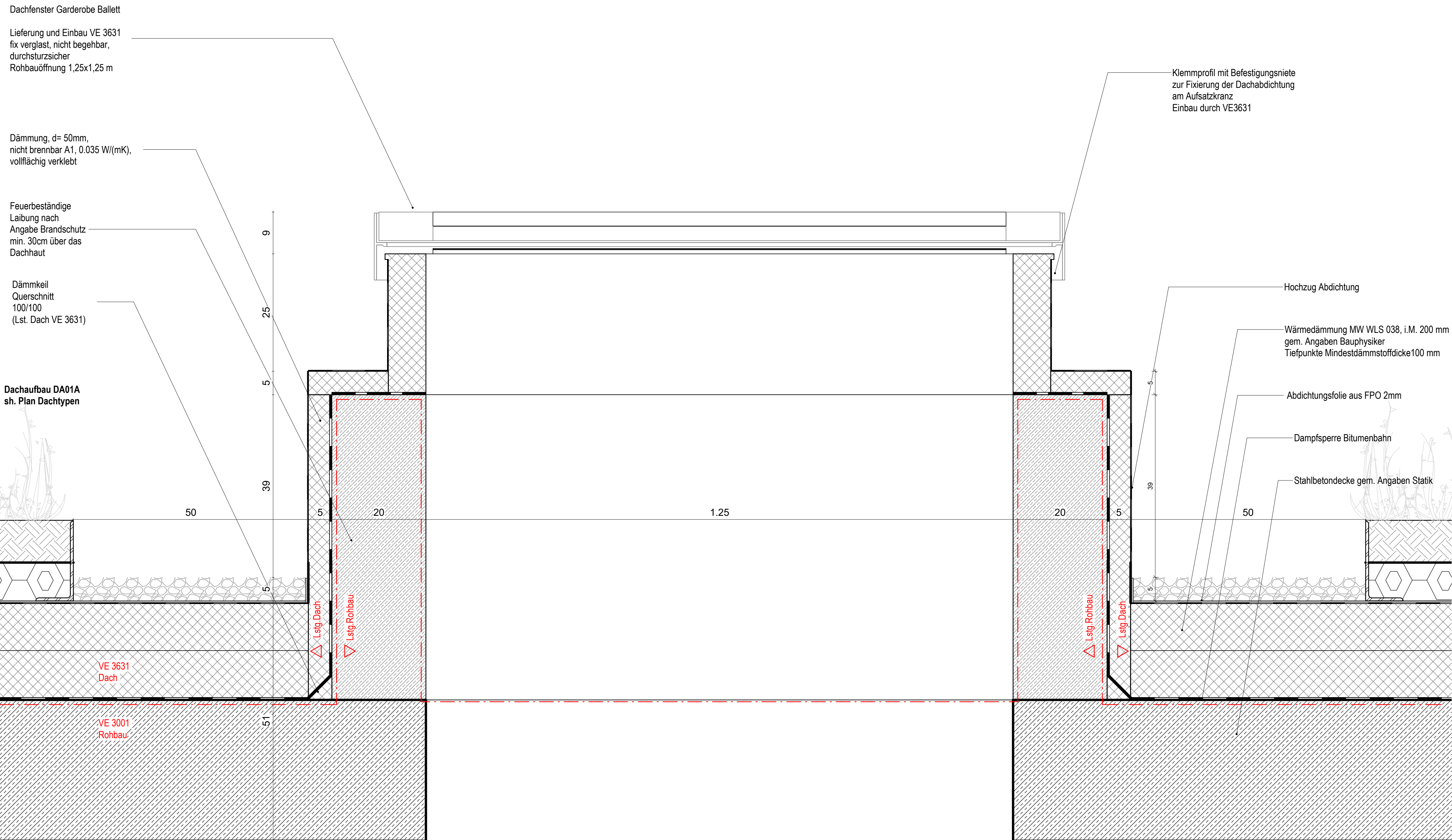
Dachfenster 1:5
